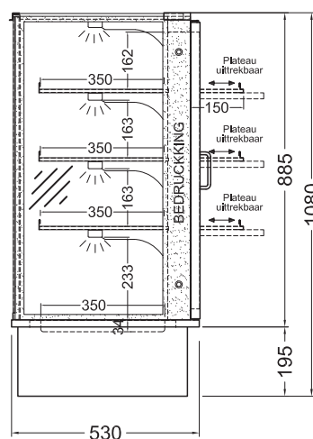
(Zijaanzicht)
